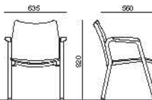
SEDIA CON POGGIA BRACCIA -
