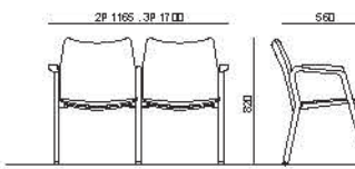
PANCA CON POGGIA BRACCIA -
